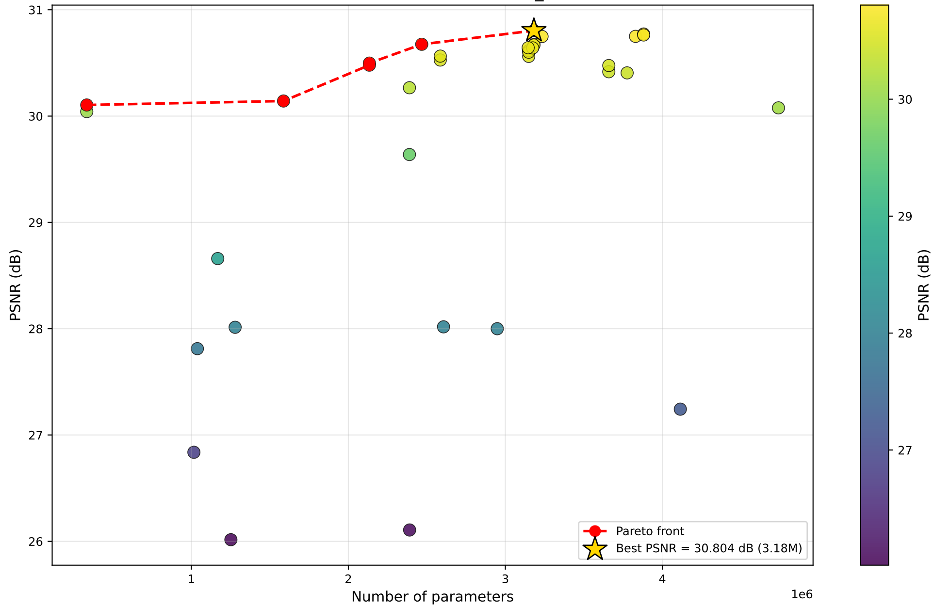
PSNR vs #Parameters — DHTCUN_baseline
